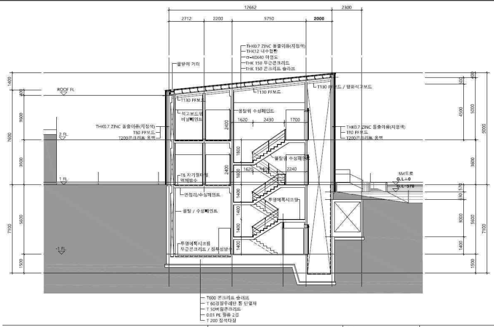
중 단면도 - 1
